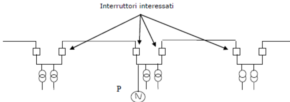
Figura E-16: Produttore connesso in antenna.
