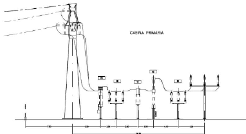
Figura E-2: Allacciamento Cliente AT Passivo in antenna da Cabina Primaria con linea AT di proprietà di Edyna (Vista laterale di dettaglio lato Cabina Primaria).
