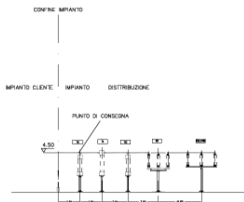
Figura E-11: Allacciamento Cliente AT Passivo in antenna da Cabina Primaria impianto adiacente alla Cabina Primaria (Vista laterale).
