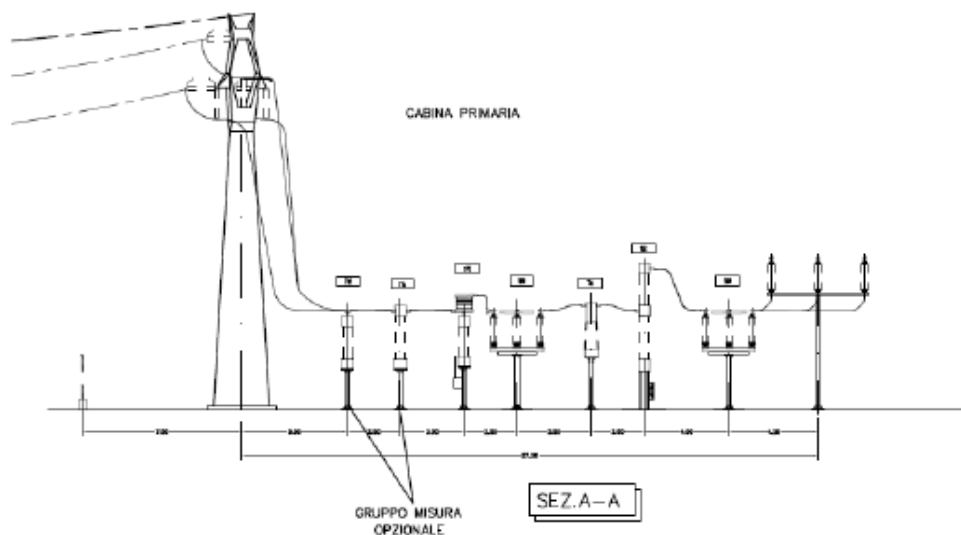
Figura E-7: Allacciamento Cliente AT Attivo in antenna da Cabina Primaria con linea AT di proprietà di Edyna (Vista laterale di dettaglio lato Cabina Primaria).
