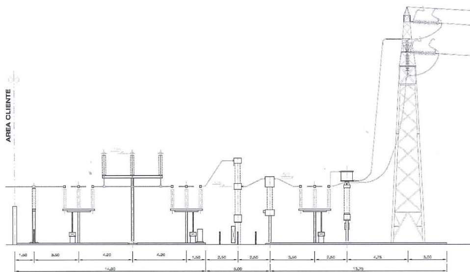
Figura E-15: Impianto di rete per la consegna in caso di connessione in entrata (Vista laterale).
