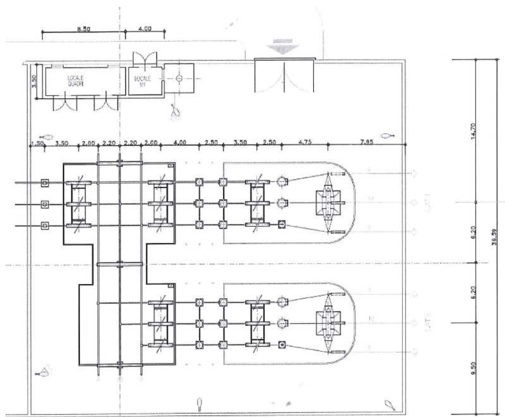
Figura E-14: Impianto di rete per la consegna in caso di connessione in entrata-esce (Vista in pianta).
