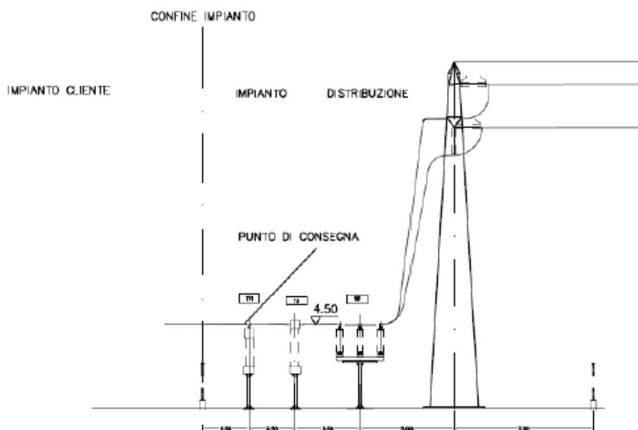
Figura E-4: Allacciamento Cliente AT Passivo in antenna da Cabina Primaria con linea AT di proprietà di Edyna (Vista laterale di dettaglio lato consegna Cliente).
