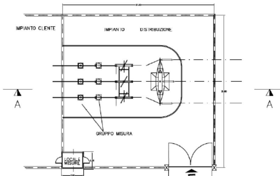
Figura E-3: Allacciamento Cliente AT Passivo in antenna da Cabina Primaria con linea AT di proprietà di Edyna (Vista in pianta dell'impianto di rete per la connessione presso il Cliente).
